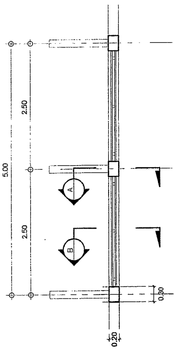
แบบแปลนหัว SCALE 1:50
